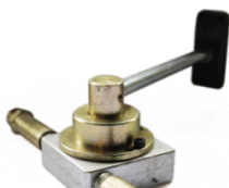
Ручка троса реверса с тросом в сборе виброплит Impulse VPR125, VPR160 DP00203
